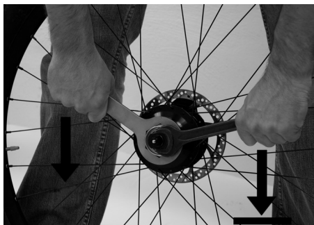
Abbildung 3: Demontage des Rohloff Lock-Rings von Rohloff SPEEDHUB 500/14
