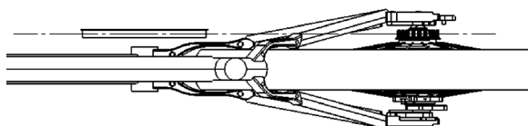
Abbildung 3: Ausrichten des Front Sprockets
