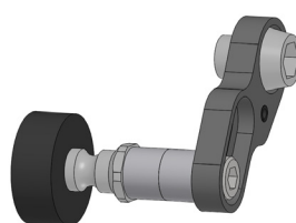
Abbildung 6: 2x Spacer
