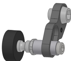
Abbildung 5: 1x Spacer
